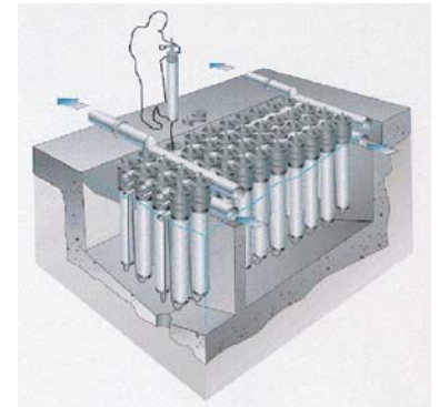
Microfiltración/Ultrafiltración sumergida (MF/UF)
